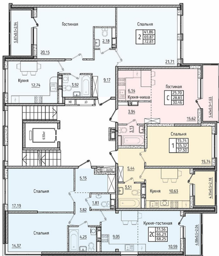
4-9 этаж - 1 секция
